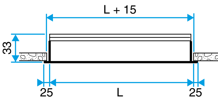
Diffuseur ALD 610 - 620
