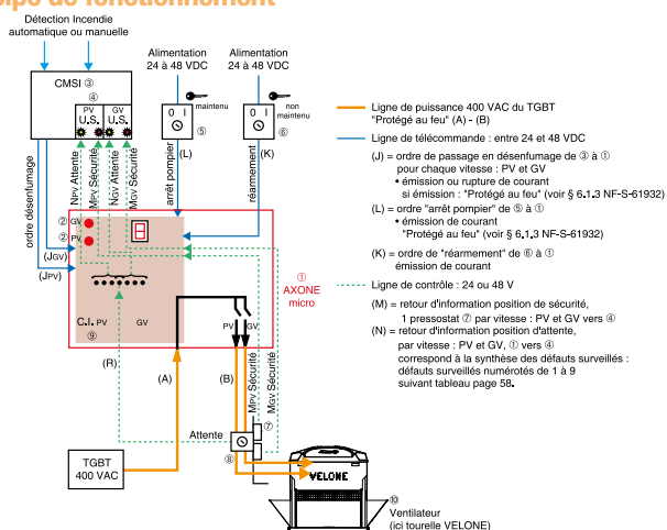
Schéma de principe d'une installation avec un coffret 2 vitesses désenfumage.
