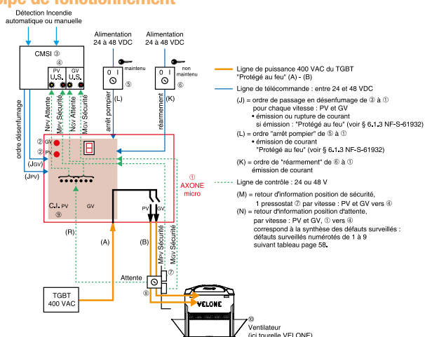
Schéma de principe d'une installation avec un coffret 2 vitesses désenfumage avec un démarrage progressif
