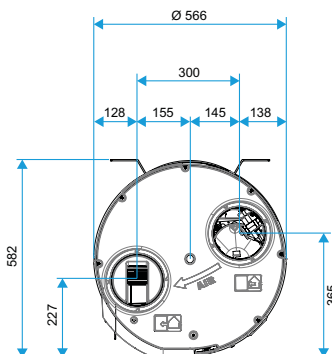
Encorement T.Flow® Hygro+ - Raccordement aéraulique
