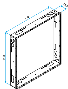
Contre-cadre OPTONE
