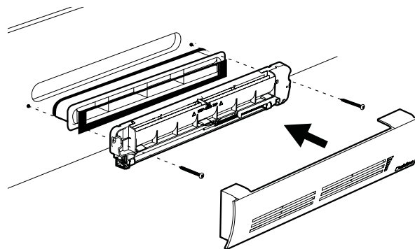
Mise en œuvre entrée d'air EHC
