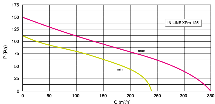
Courbe aéraulique XPro 125
