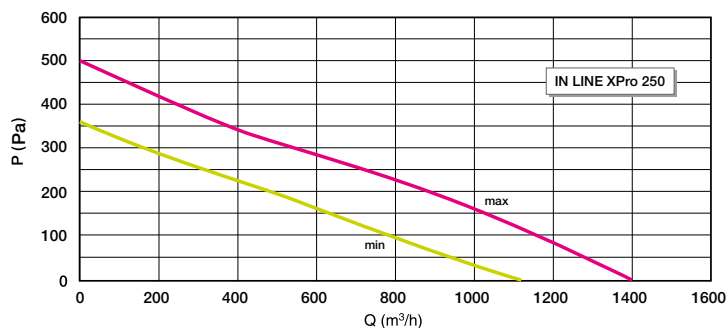
Courbe aéraulique XPro 250
