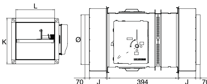
Encombrement ISONE®2.1 GM
