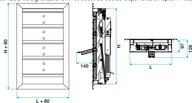
Encombrement (mm)
