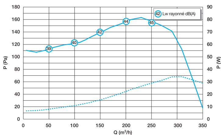
Courbes aérodynamique, de consommation et valeurs acoustiques EasyHOME HYGRO COMPACT MP
