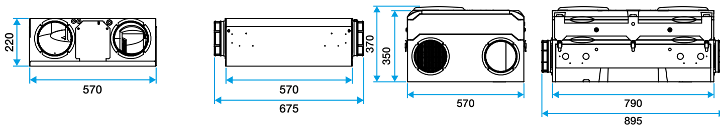
Moto-ventilateur
