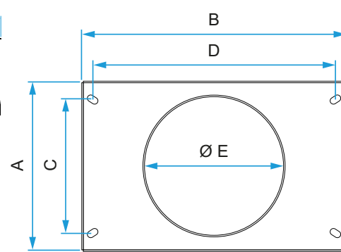
Pièce de transformation rectangulaire &gt; circulaire VEX400
