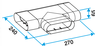
Té 90° horizontal
