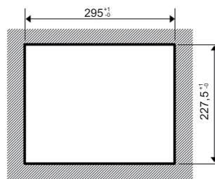
Schéma des dimensions de découpe du panneau
