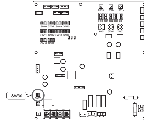
Cartes de circuits imprimés de l'interface de l'unité principale
