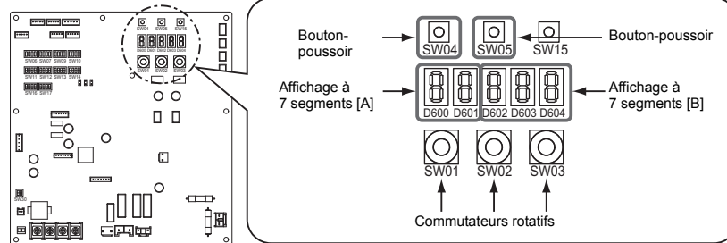
Carte de circuits imprimés de l'interface
