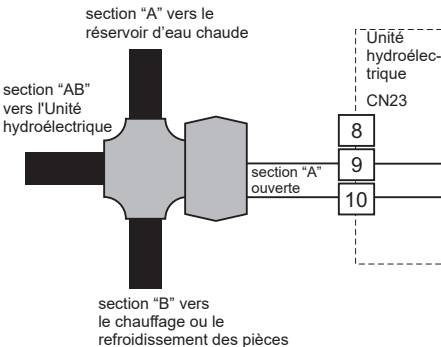
▼ Fig.7-24 Type 1 RETOUR DU RESSORT
