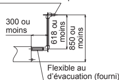
Dimensions de l'installation d'évacuation
