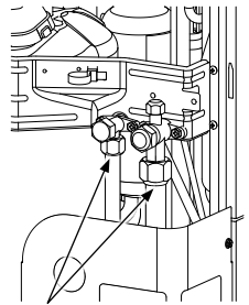
Tuyau latéral de l'unité intérieure
