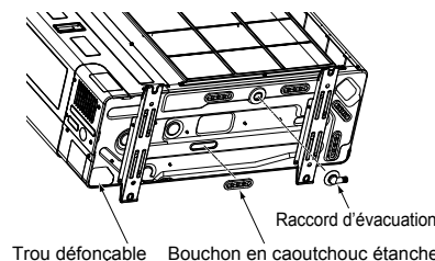
Bouchon en caoutchouc étanche (5 pièces)
