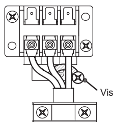
Câble de raccordement (Unité C)
