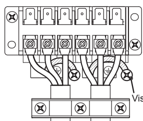
Câble de raccordement (Unité C)
