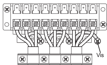
Câble de raccordement (Unité C)
