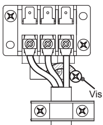
Câble de raccordement (Unité C) * Exemple de raccordement (RAS-3M26U2AVG-E)
