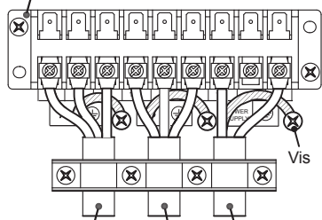
Câble de raccordement (Unité A) Câble d'alimentation Câble de raccordement (Unité B)
