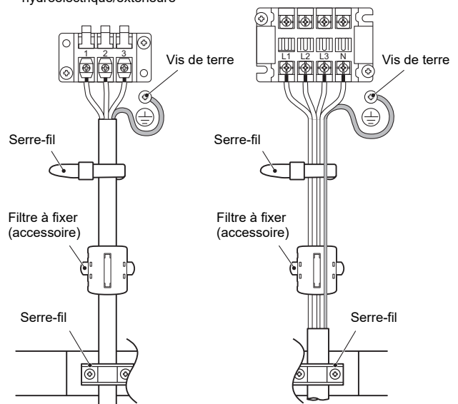
Câble de raccordement des unités hydroélectrique/extérieure
