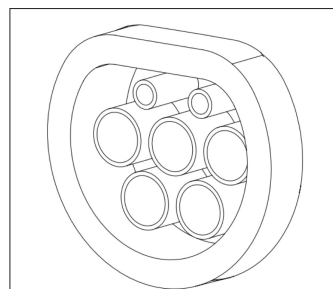
IEC 62196-2 2. típus - szüllyesztett változat
