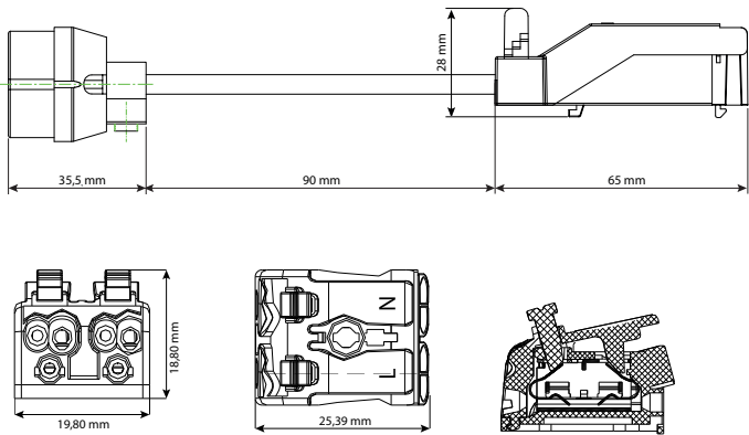
Schémas techniques
