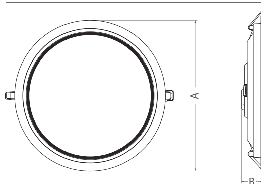
Schéma technique
