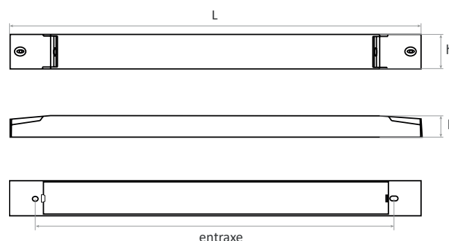
Schémas techniques
