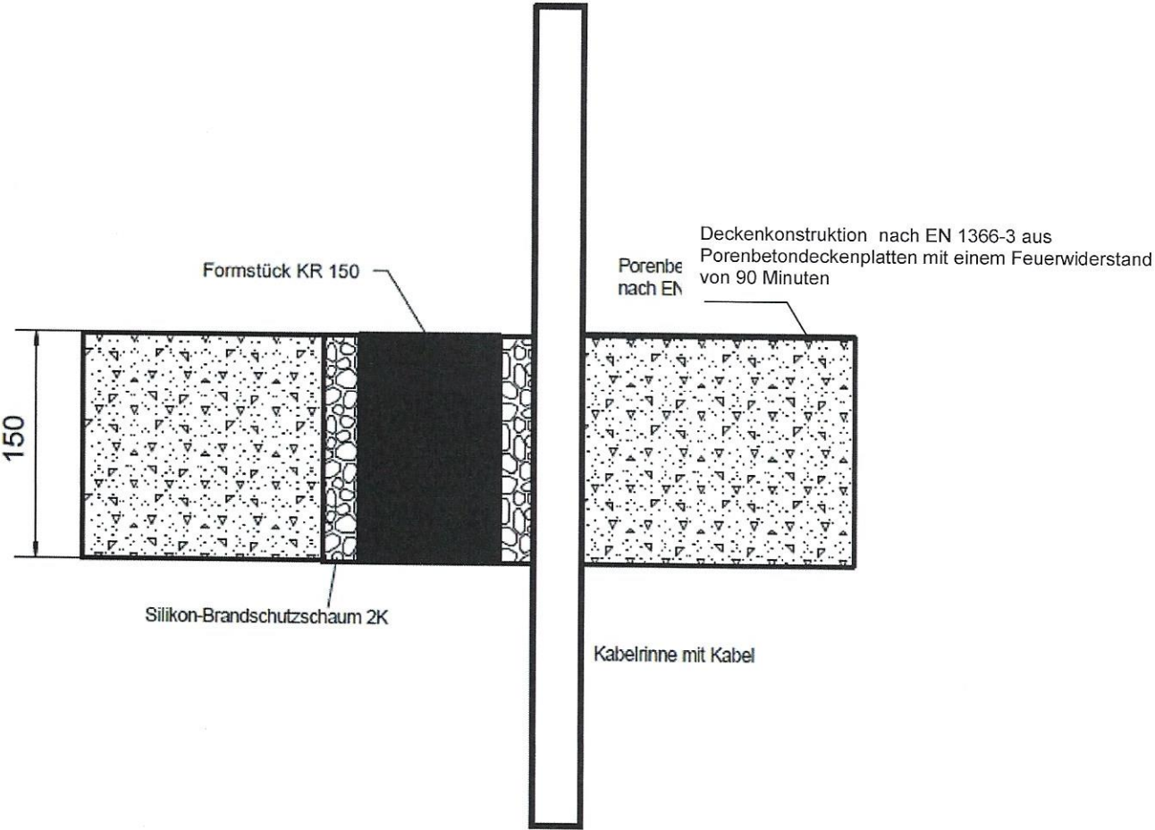
Bausatz aus "Silikon-Brandschutzschaum 2K" und "Formstück KR 150"
