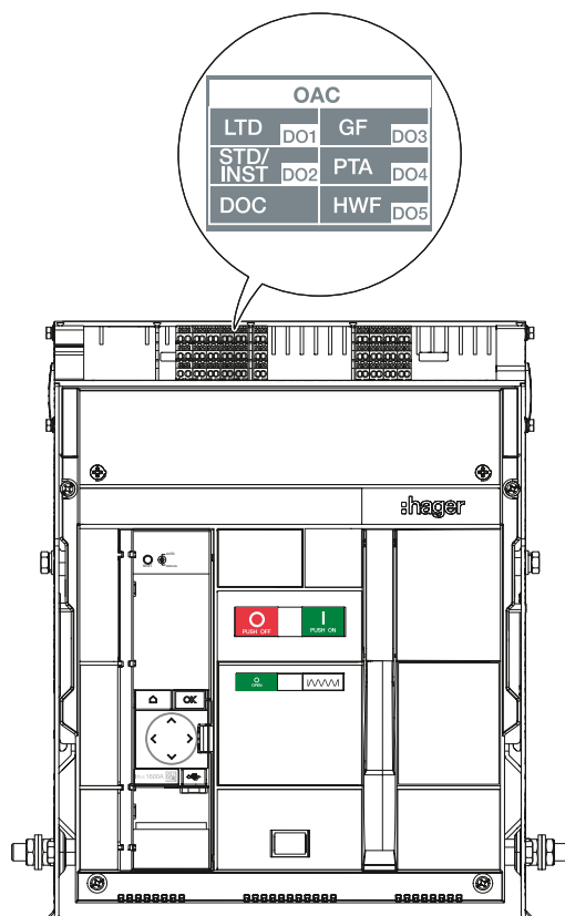
Disjoncteur fixe
