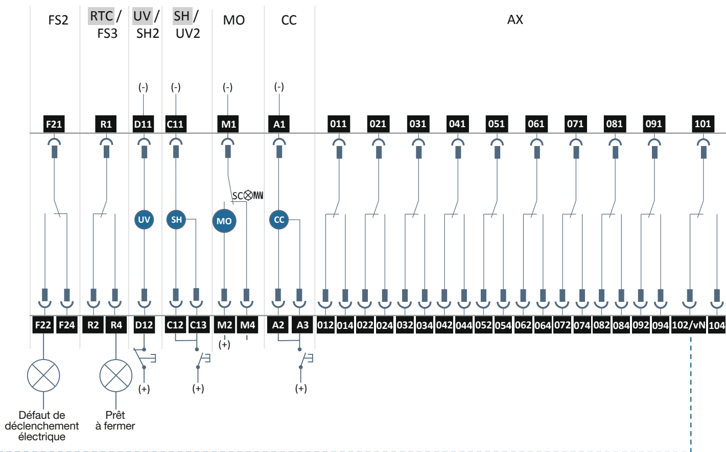
Schéma électrique du contact de défaut de déclenchement FS3, de la bobine à émission SH2 et de la bobine à manque de tension UV2.
