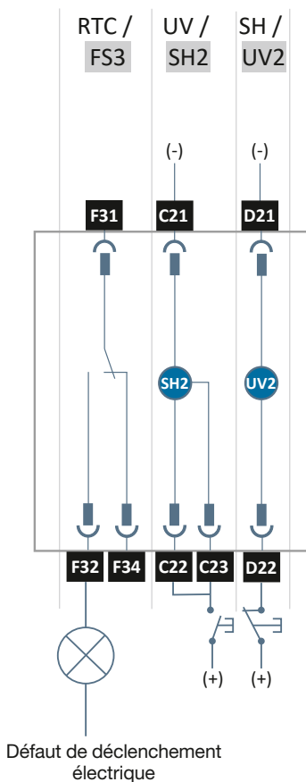
Schéma électrique du contact de défaut de déclenchement FS3, de la bobine à émission SH2 et de la bobine à manque de tension UV2.
