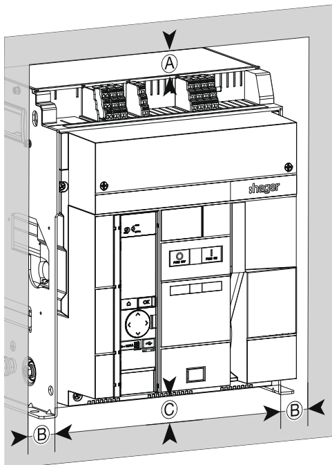
Disjoncteur fixe
