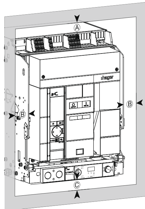
Disjoncteur débrochable
