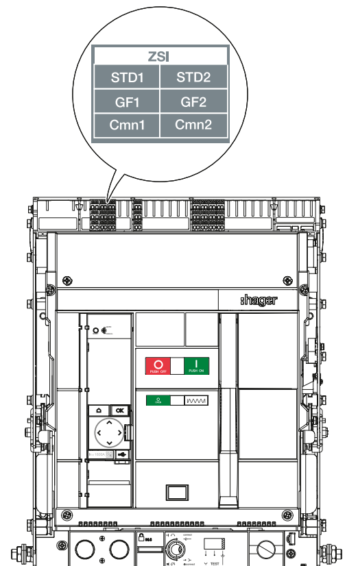
Disjoncteur débrochable
