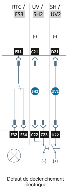
Schéma électrique du contact de défaut de déclenchement FS3, de la bobine à émission SH2 et de la bobine à manque de tension UV2.
