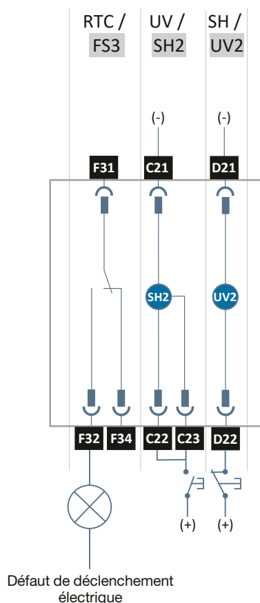
Schéma électrique du contact de défaut de déclenchement FS3, de la bobine à émission SH2 et de la bobine à manque de tension UV2.
