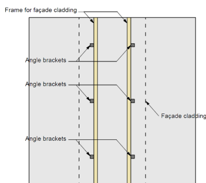
Figure 1.2 - Exemple de fixation statistiquement indéterminée pour un ancrage
