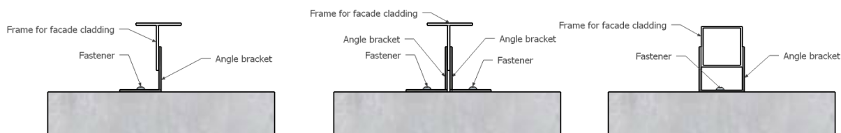
Figure 1.1- Connection de revêtements de façade dans des blocs de maçonnerie
