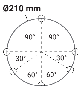
Schéma de pré-perçage de fixation
