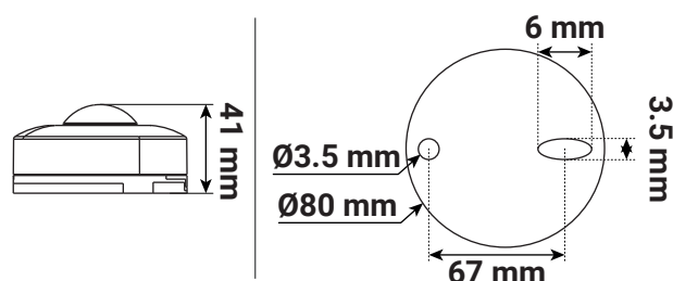
Schéma de fixation
