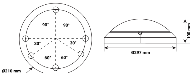
Schéma de pré-perçage de fixation
