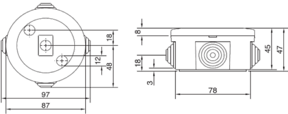
Pico BDD Ø 80
