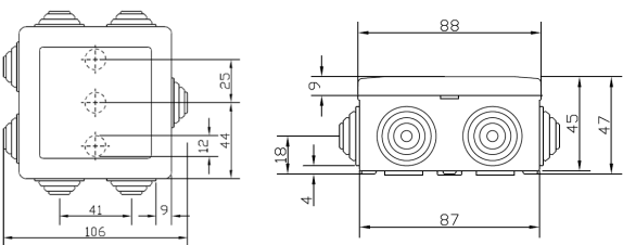
Pico BDD 80x80
