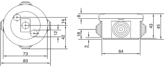
Pico BDD Ø 60
