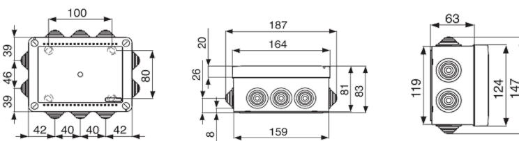
Pico BDD 150x110
