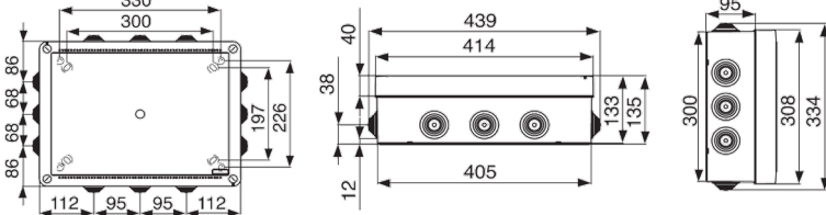
Pico BDD 380x300
