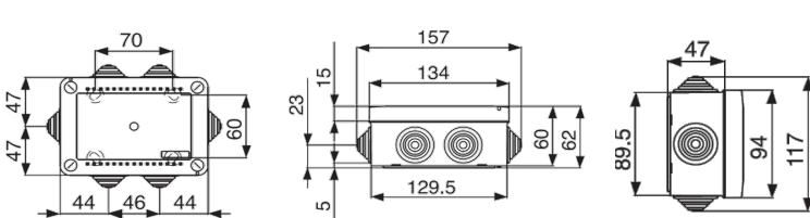
Pico BDD 120x80
