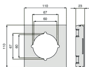
CSA-60 Entraxe 60
