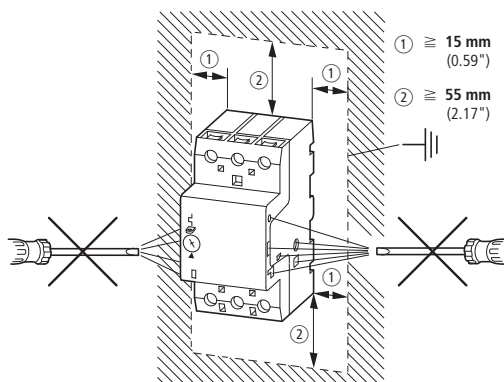
Abbildung 6: Montage PKZM0-.../XTPR...BC1NL und PKZM0-...-T/XTPT...BC1NL
