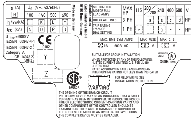
Abbildung/Figure 9: Typenschild/Rating plate PKZM0-.../XTPR...BC1NL, PKZM0-...-T/XTPT...BC1NL
