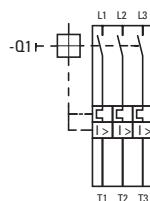
Abbildung 2: Schaltbild Motorschutzschalter PKZM0-.../XTPR...BC1NL und PKZM0-...-T/XTPPT...BC1NL
