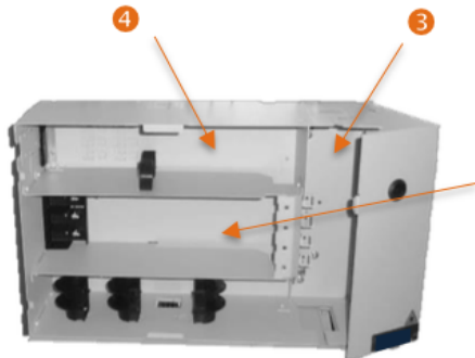
Coffret abonnés 12 à 48 logements IC5752
