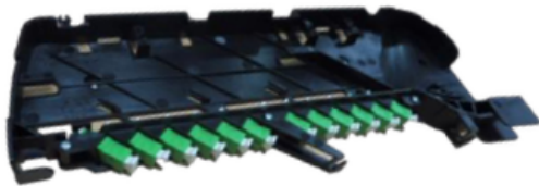
Module 12 raccords pour câble pré-connectorisé IC5754
