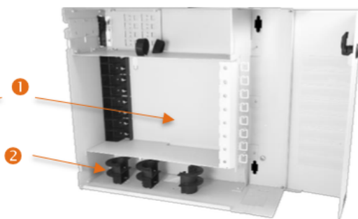
Coffret abonnés 49 à 96 logements IC5951
