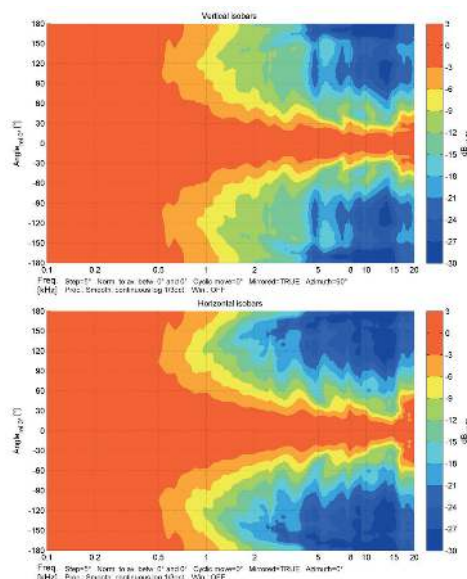
Diagrammes polaires
