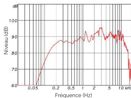
Bande passante
