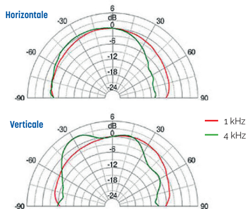
Directivité
