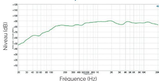
Bande passante
