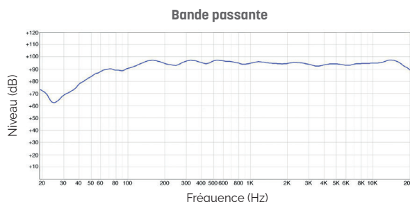
Bande passante
