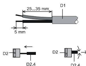
figure 5: Brancher / Débrancher le câble bus
