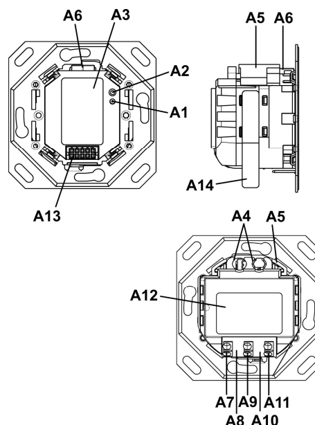
figure 2: Emplacement / fonction des éléments d'affichage et de commande
