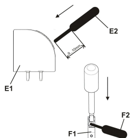
figure 6: Branchement / débranchement des circuits d'alimentation et de charge
