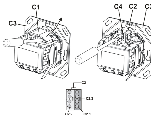
figure 4: Connecter / Déconnecter le bornier bus
