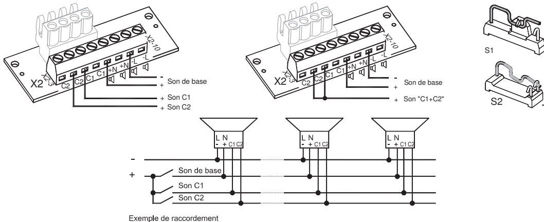
Exemple de raccordement
