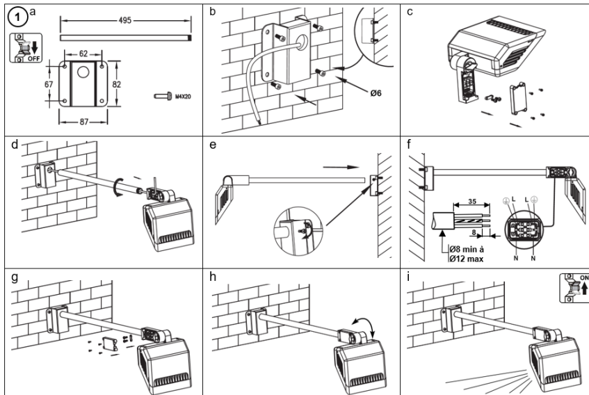
o Fig. 1 : Fixation murale sur tige non fournie (0887 – Fixation FA57 Blanc ou 0878 – Fixation FA57 Noir)
