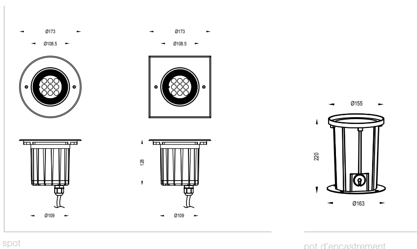
pot d'encastrement
