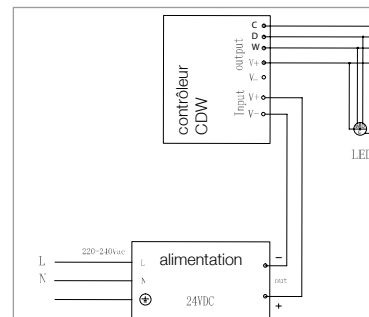
câblage CDW
