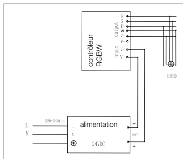
câblage RGBW
