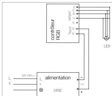
câblage RGB
