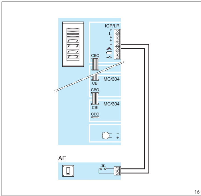
Fig.16-17 Schema di collegamento del pulsante ausiliario apriporta (AE).
