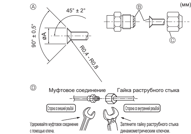
А Раструбный стык - размеры Б Момент затяжки гайки раструбного стыка Fig. 4-1
