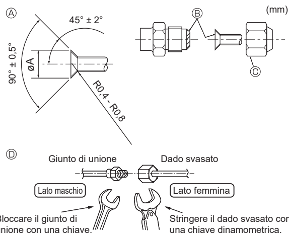
Ⓐ Dimensioni di taglio per raccordo a cartella Ⓑ Coppia di serraggio del dado a cartella
