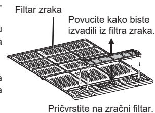
Pričvrstite na zračni filtari.
