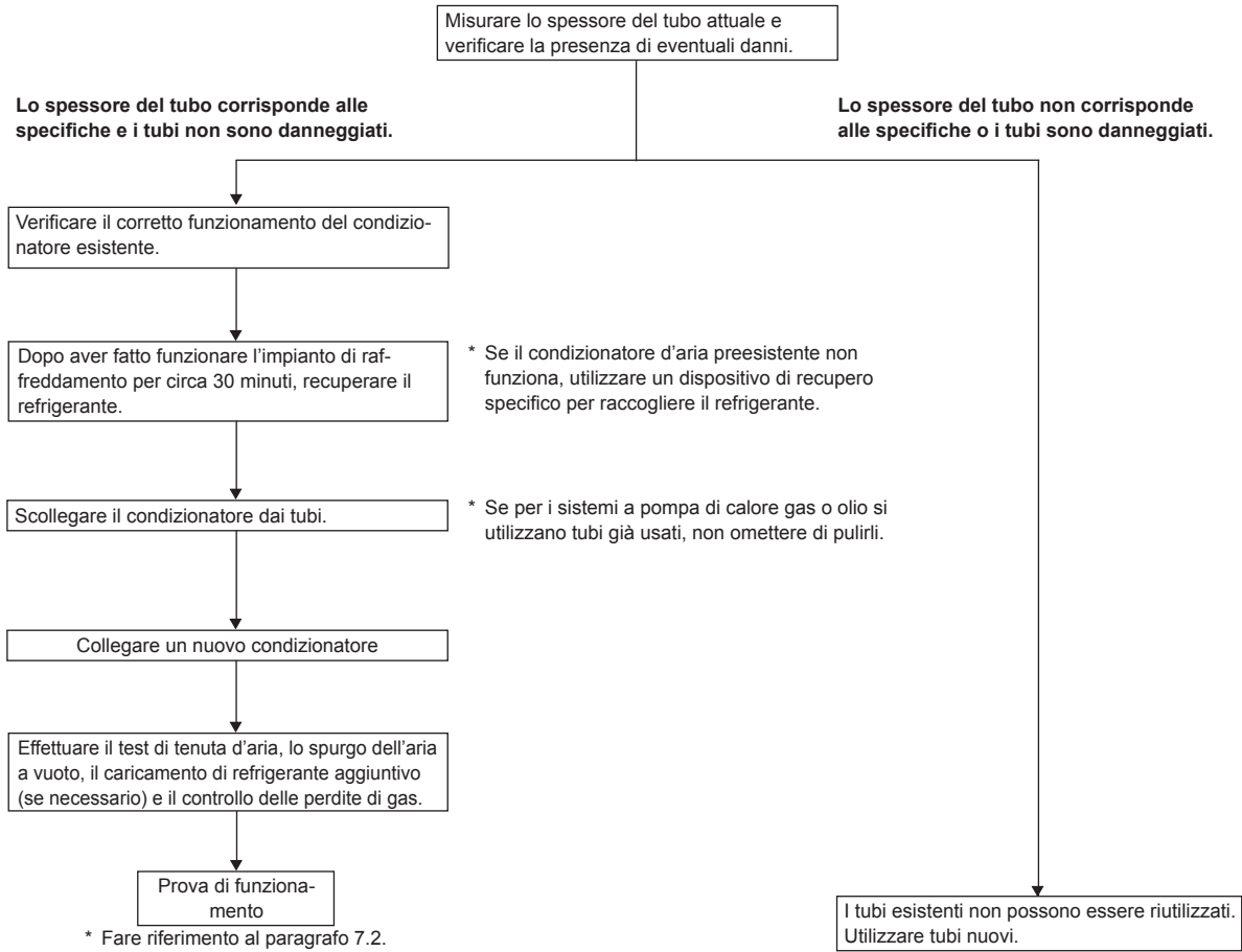
<Limiti dell'installazione della tubazione del refrigerante>
