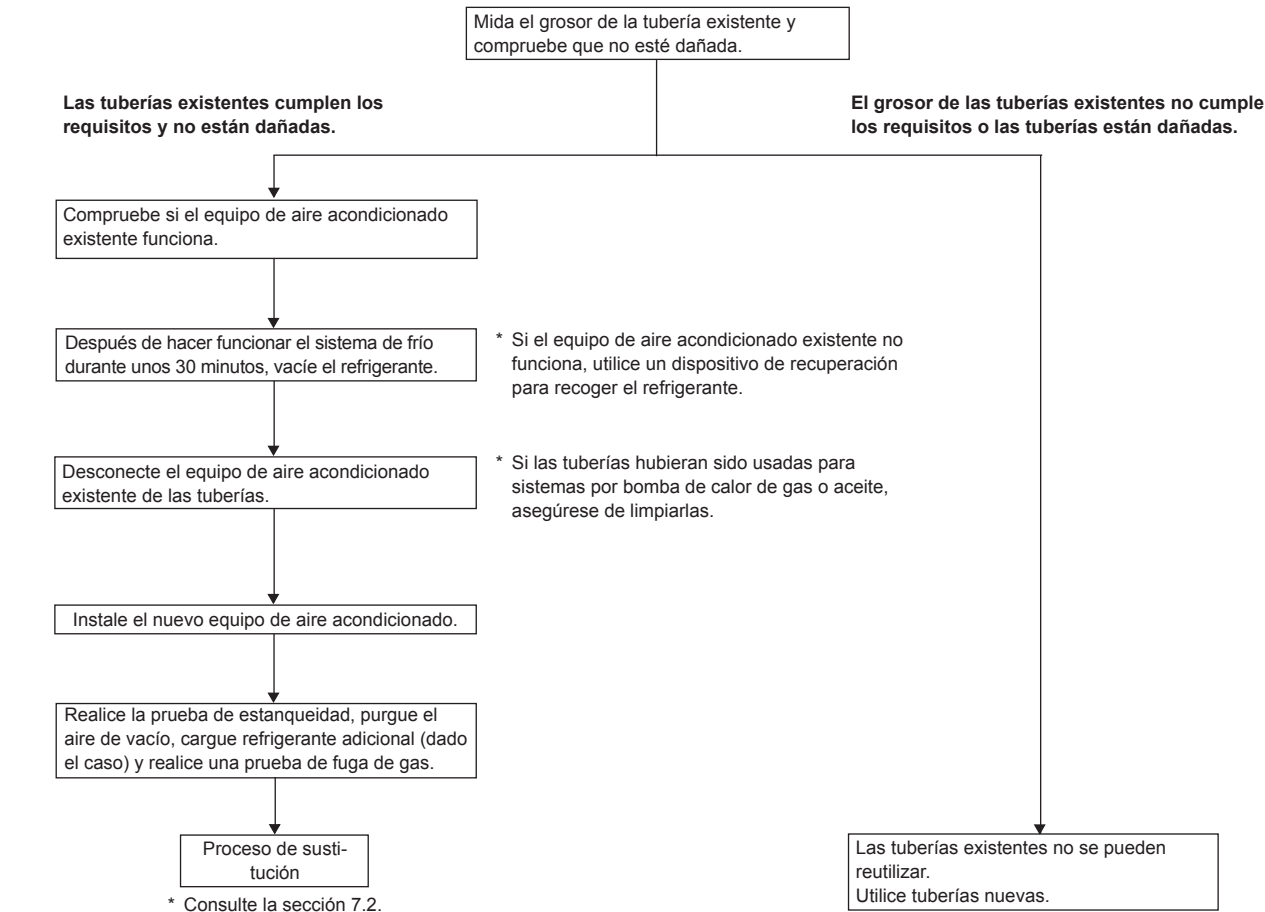
<Límites de la instalación de tubos de refrigeración>
