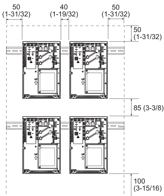
Installation sur un rail DIN
